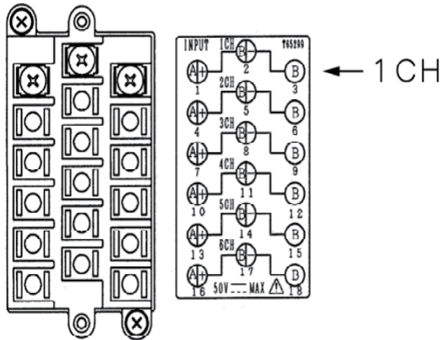
端子図
