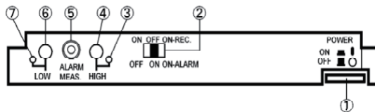
前面パネル（警報上下限設定用）
