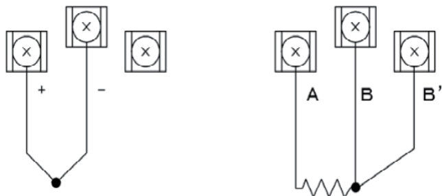
入力配線（熱電対入力）
