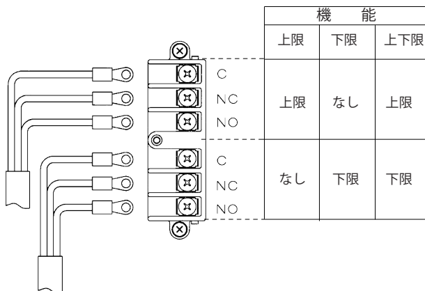
警報出力端子の配線
