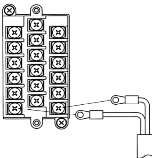
チャートロック用制御端子の配線
