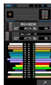
CRI 比較
